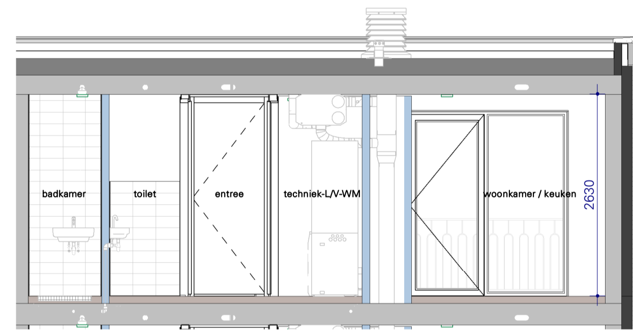
VK Doorsnede B - Blok E -bnr110
