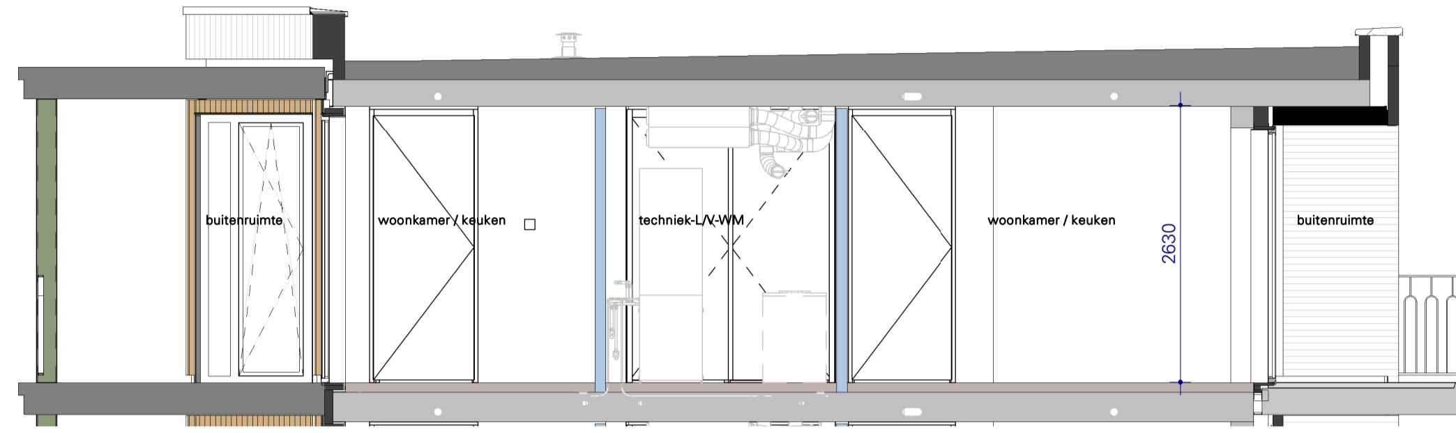
VK Doorsnede A - Blok E -bnr110
